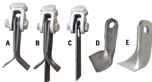
(A) - Mlatilica "Y" za usitnjavanje debljine 4 mm
