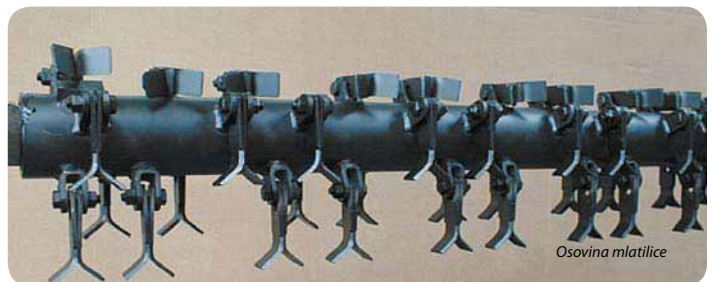
Trostruko preklapanje mlatilica uz dinamičko balansiranje.
