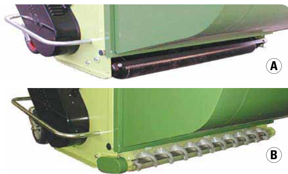
Valjak za čišćenje sa strugajućom metalnom šipkom (A) ili sa četkom za sportske terene (B)
