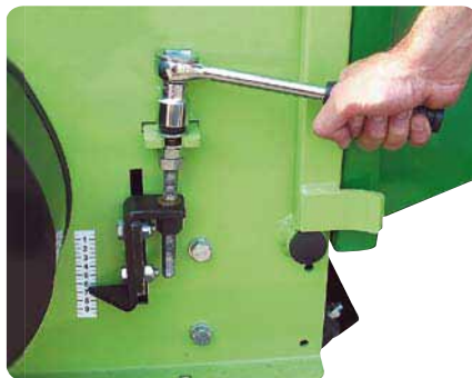
Jednostavno (milimetarsko) podešavanje visine valjka.
